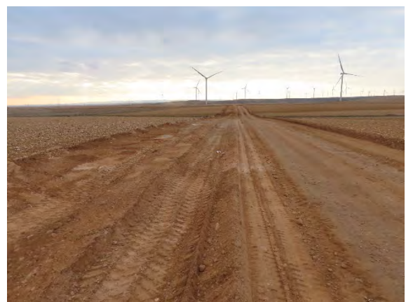
Zanja eléctrica entre los aerogeneradores REA-03 y REA-04 ya cerrada, el camino de servicio será desmantelado al finalizar la obra.
