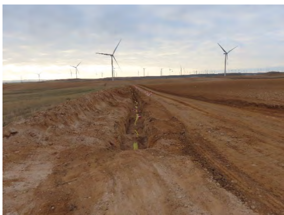
Zanja eléctrica entre los aerogeneradores REA-03 y REA-04 abierta en terreno de cultivo, con separación de suelo fértil.
