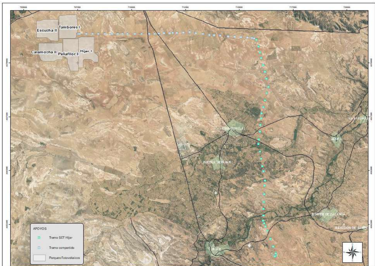
Figura 4: Emplazamiento de la LAAT 132 kV SET "Almochuel" - SET "Híjar" sobre ortofoto.
