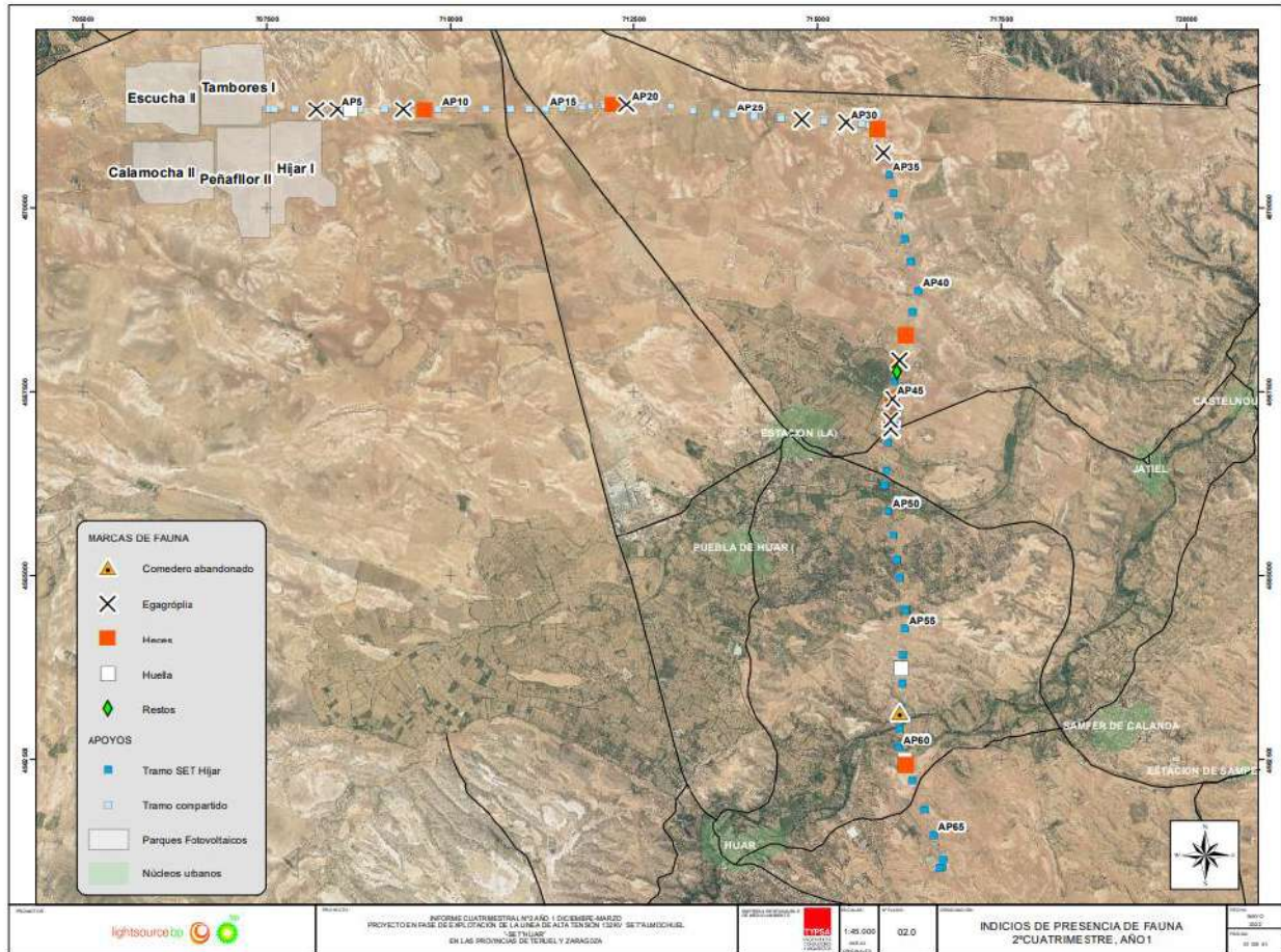
Figura 5: Plano del uso de la estructura de los apoyos e indicios de fauna bajo el bando de ancho de la línea eléctrica SET "Almochuel" SET "Híjar".
