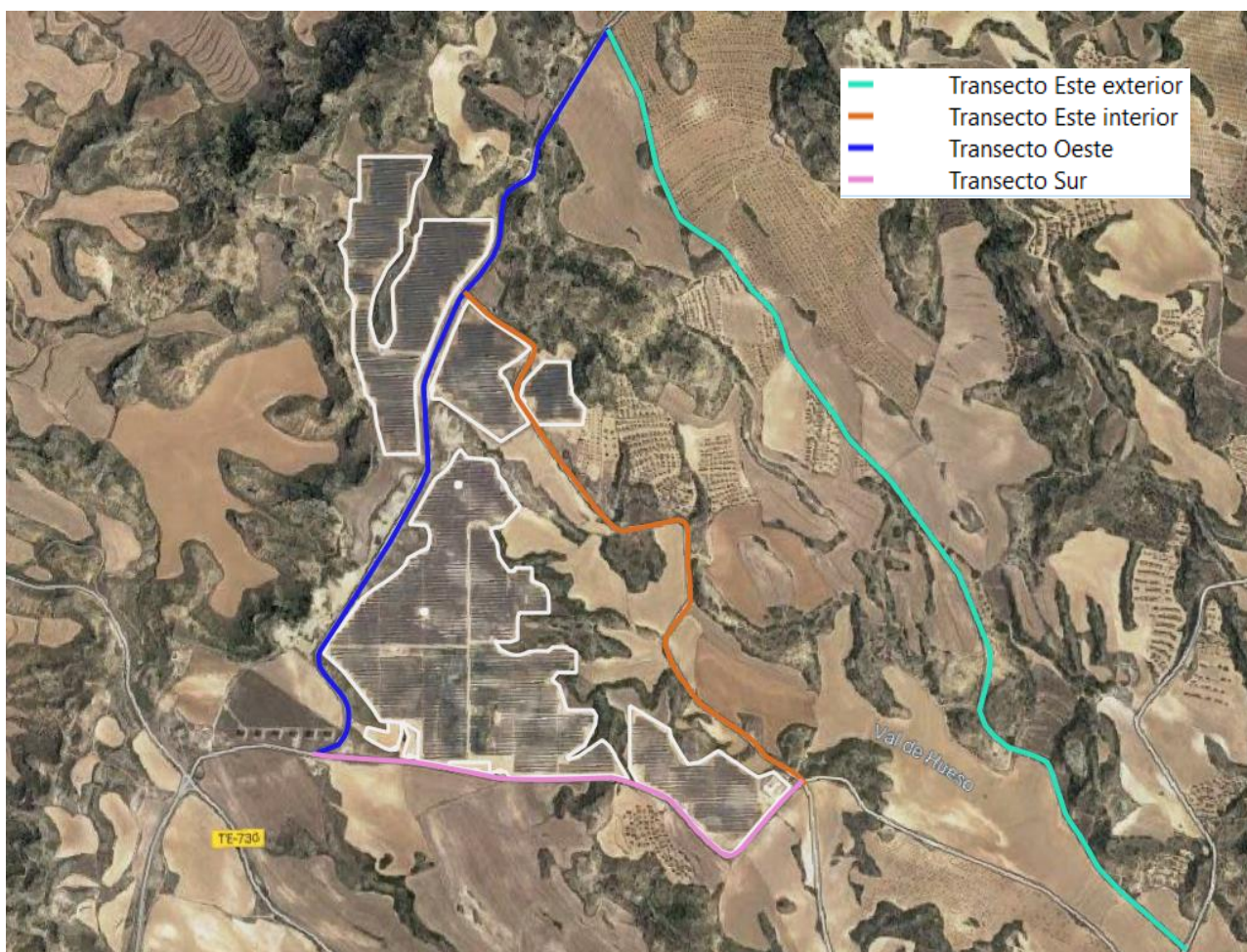
Figura 5: Transectos prospectados alrededor de la PFV
