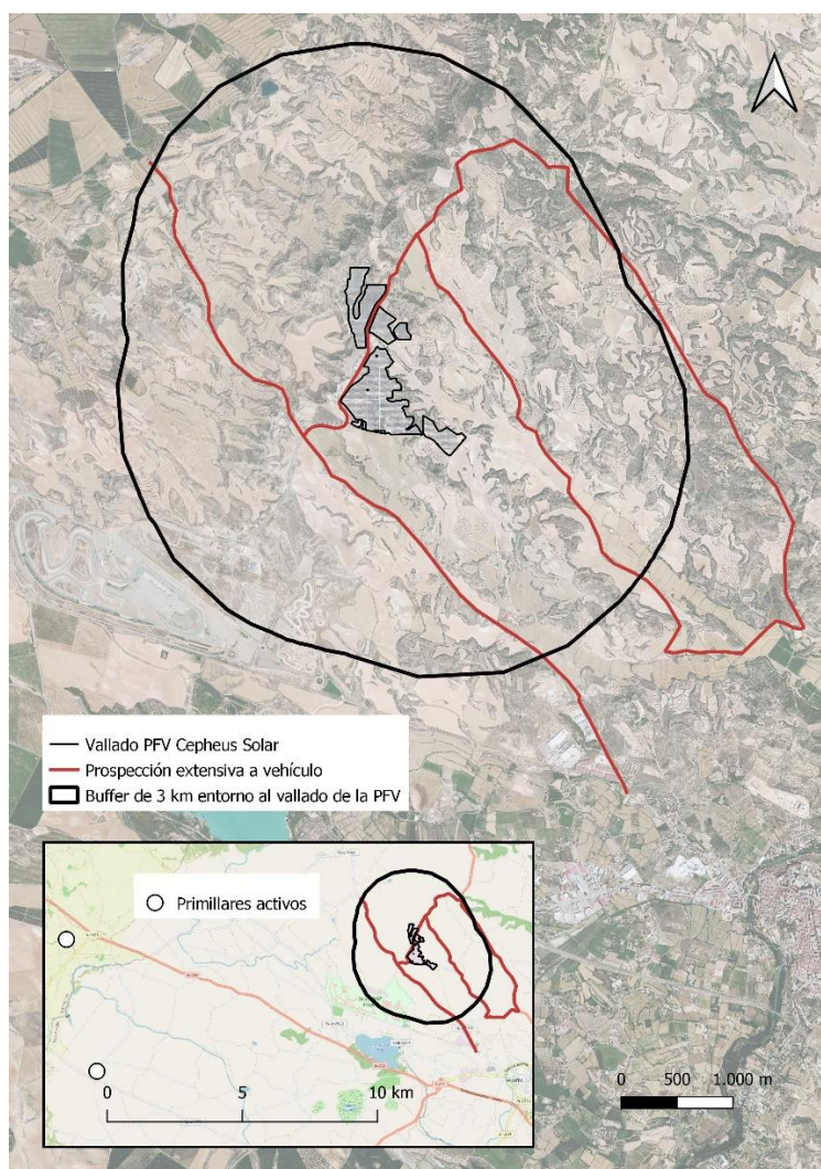
Figura 6. Prospección extensiva en vehículo y situación de las colonias más próximas de cernícalo primilla
