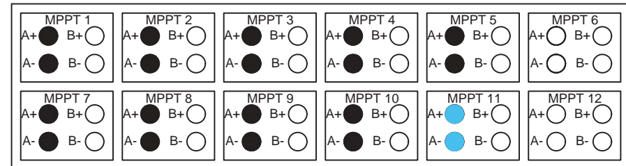
INVERSOR STR250
