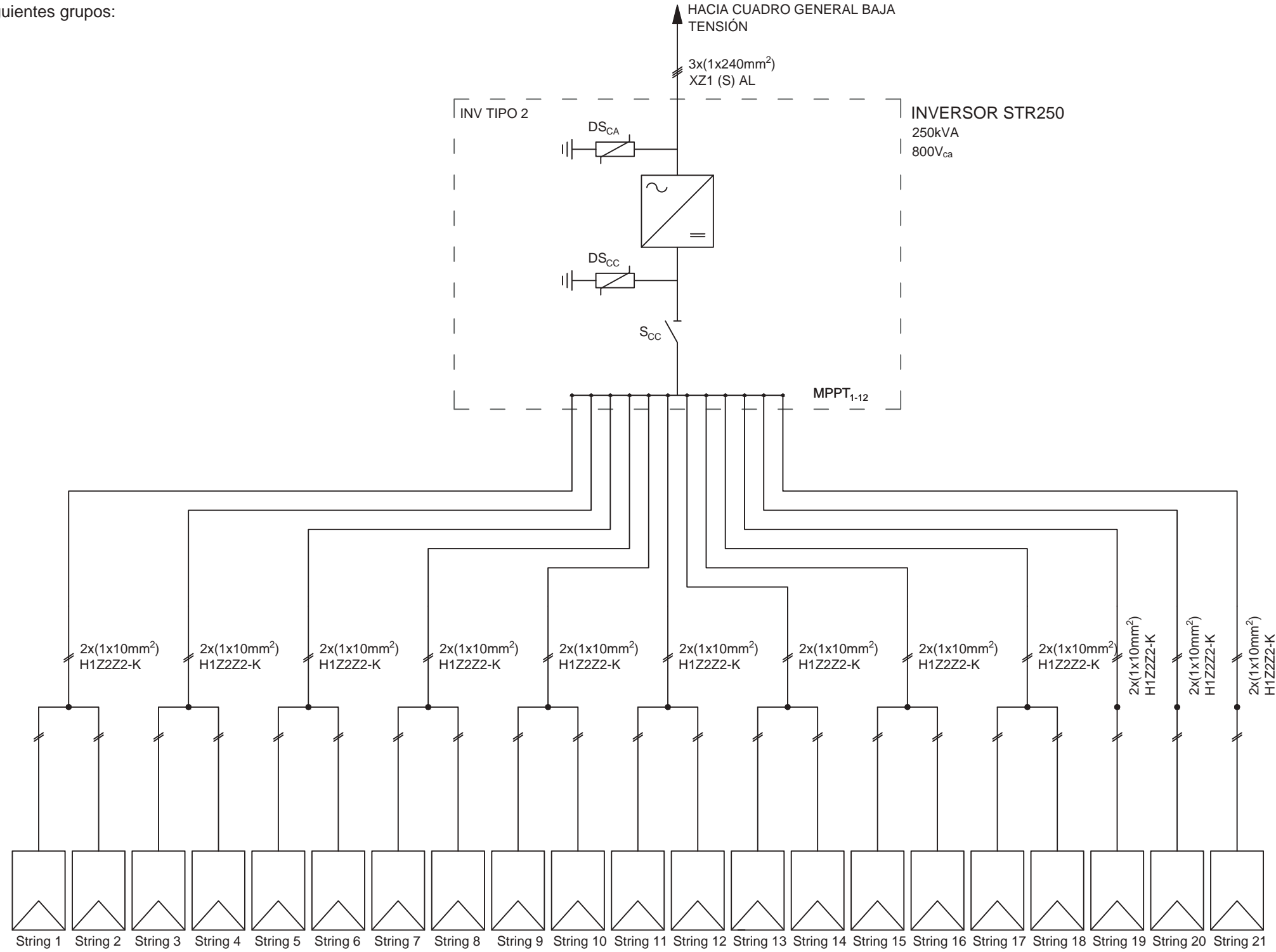
INVERSOR STR250
