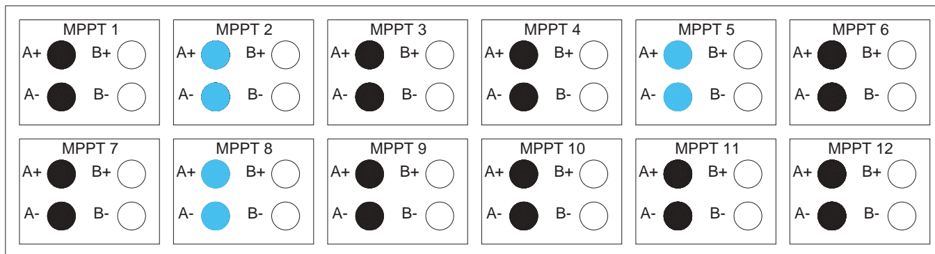
INVERSOR TIPO 6 (STR250)
