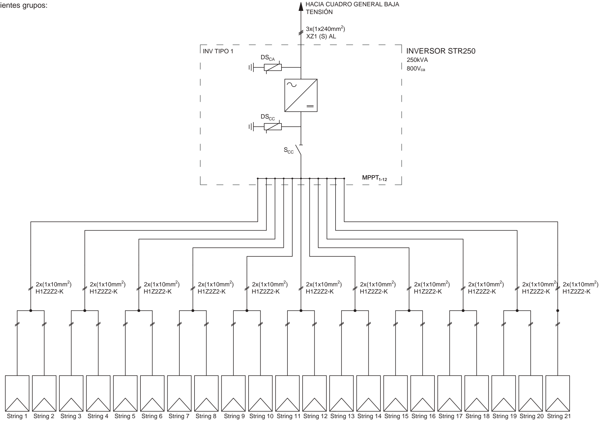
INVERSOR STR250
