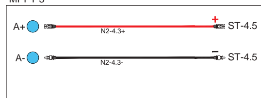
MPPT 3
