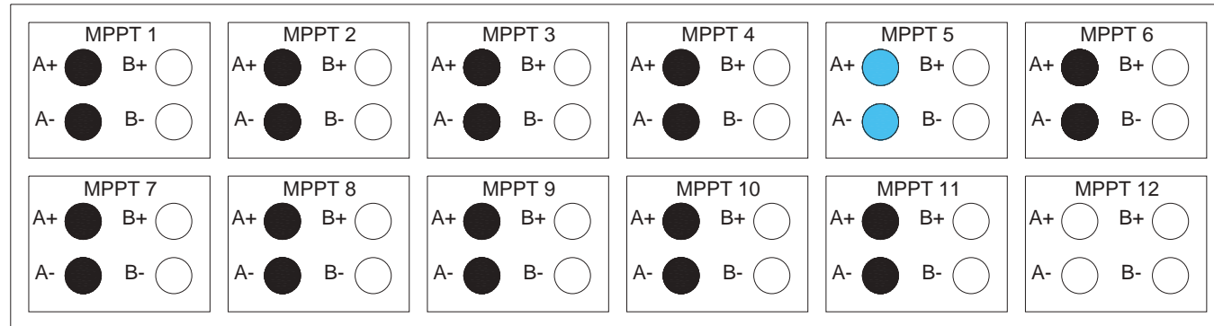
INVERSOR TIPO 1 (STR250)
