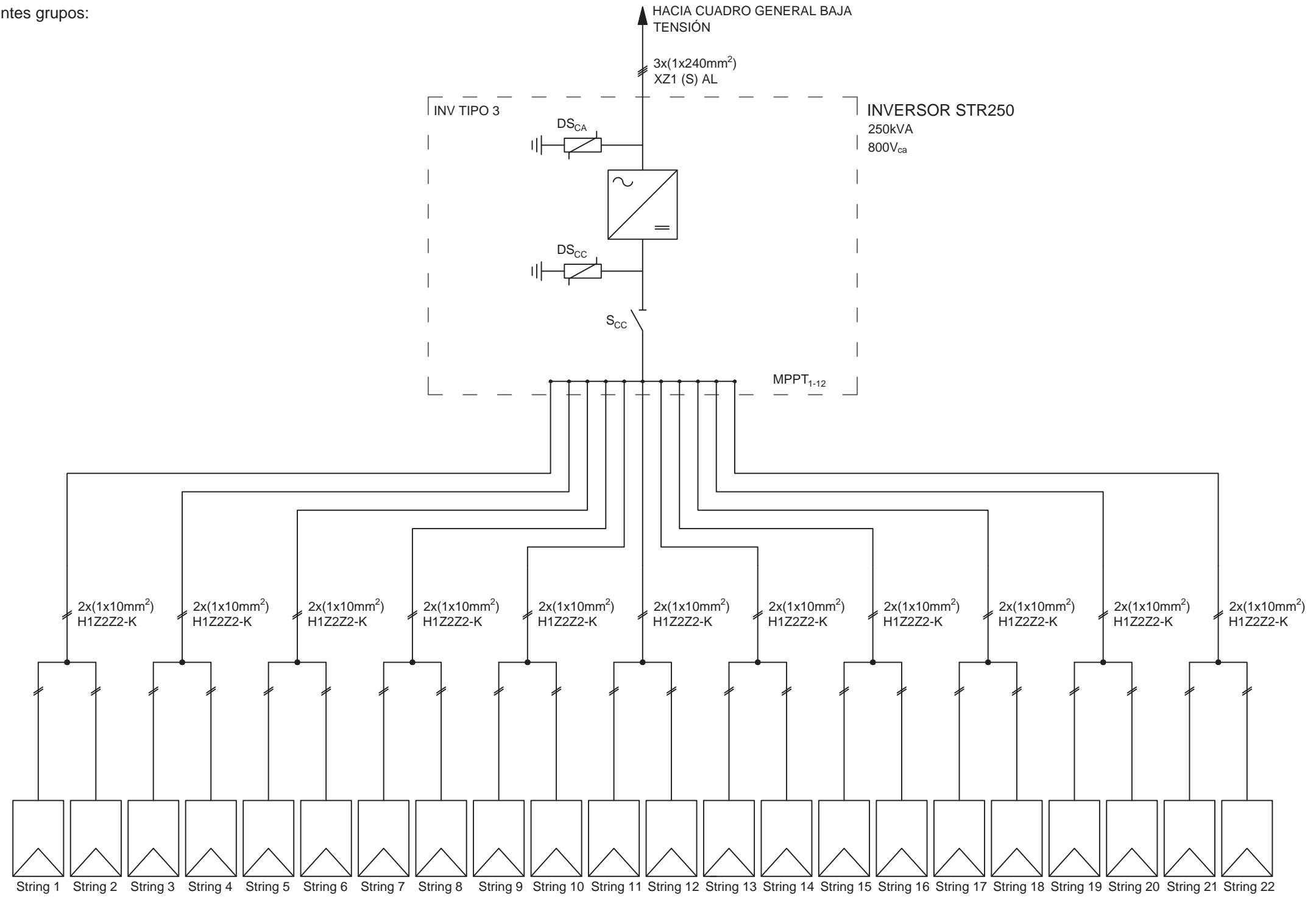
INVERSOR STR250
