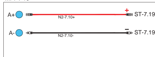
MPPT 10
