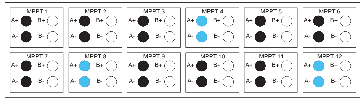
INVERSOR TIPO 2 (STR250)
