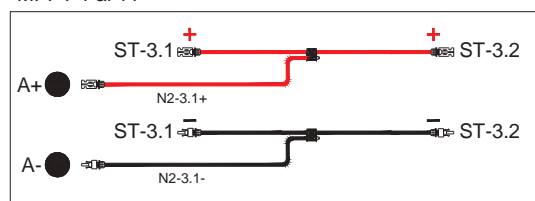
MPPT 1 al 11
