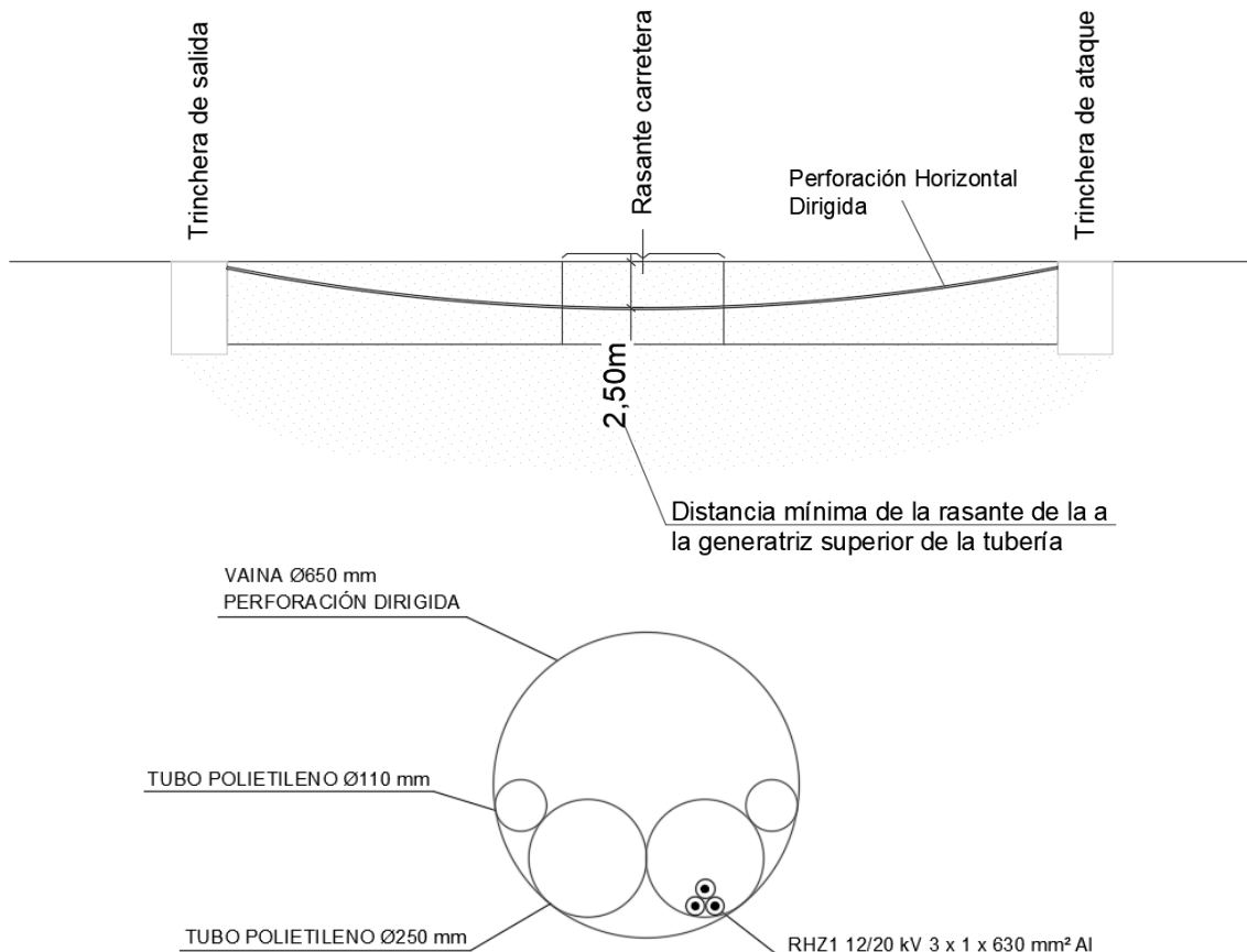
Ilustración 1. Perforación dirigida para cruzamiento de carretera
