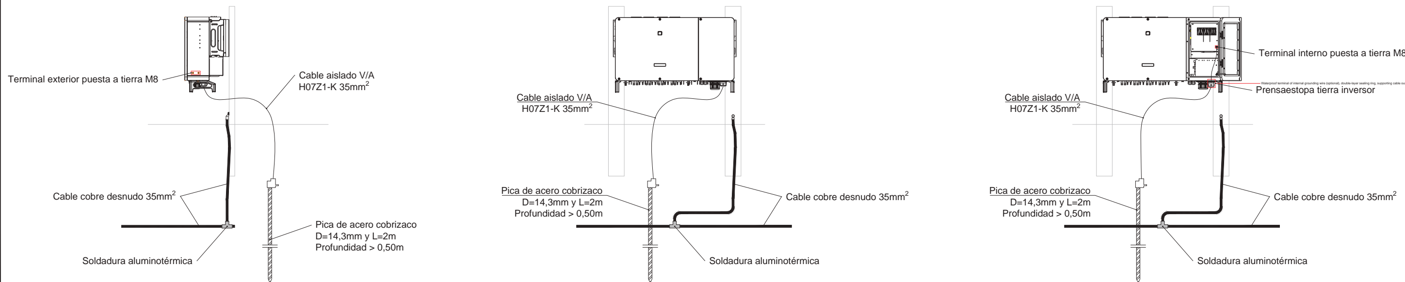
DETALLE DE TOMA DE TIERRA EN INVERSOR DE STRINGS
