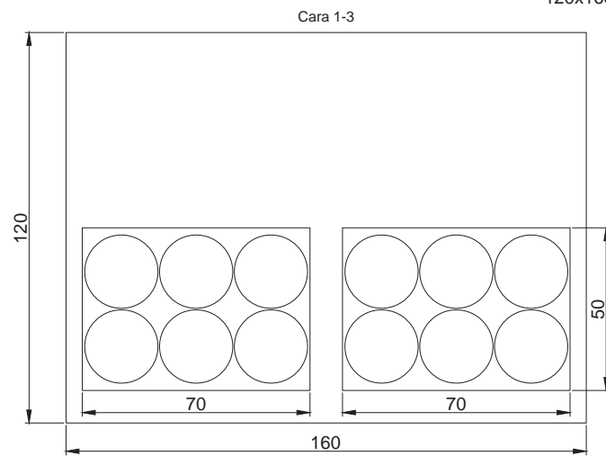
ARQUETA CT 120x160x120
