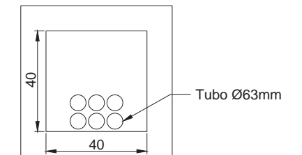
ARQUETA STRING 40x40x40
