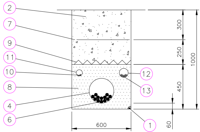
ZANJA PARA 6 CIRCUITOS BAJA TENSION EN ZONA DE TIERRA
