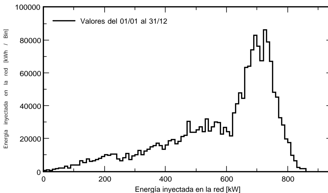
Distribución Potencia de Salida del Sistema
