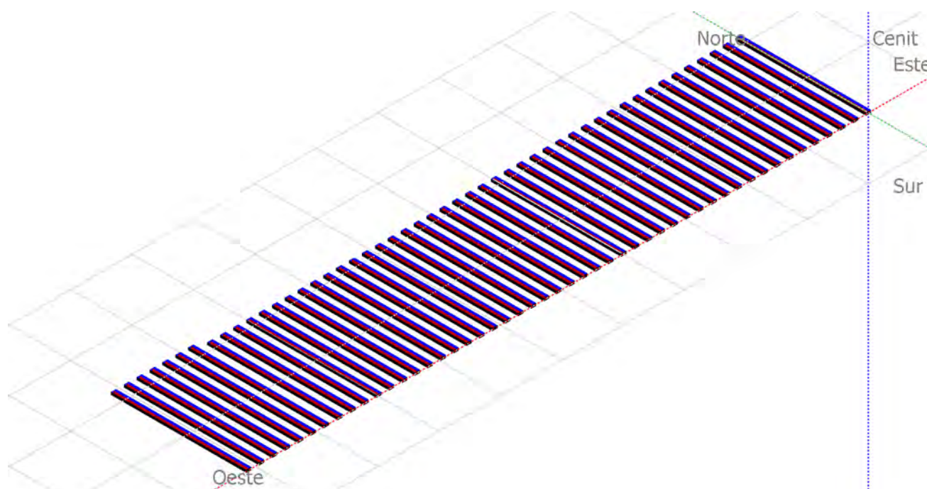
Perspectiva del campo FV y la escena de sombreado circundante
