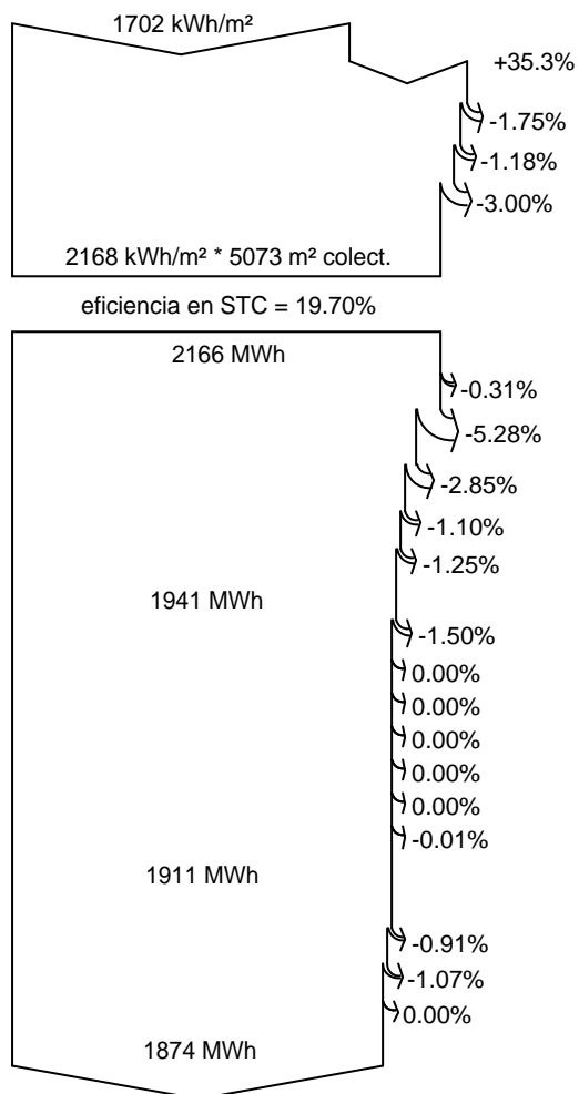
Diagrama de pérdida durante todo el año
