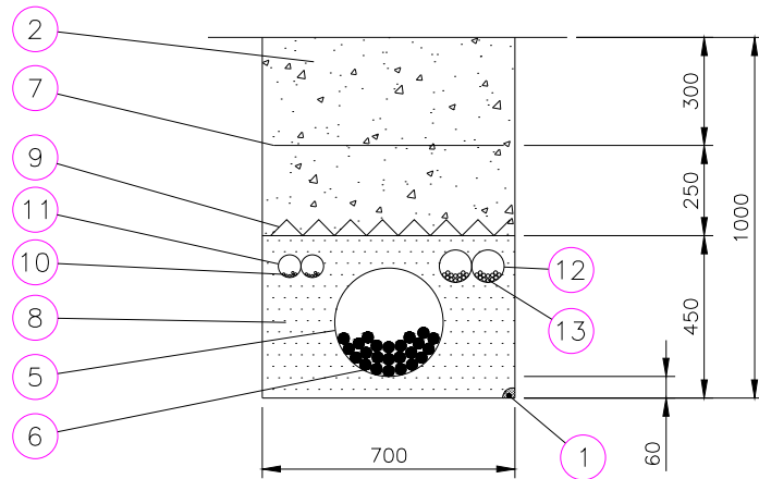
ZANJA PARA 12 CIRCUITOS BAJA TENSION EN ZONA DE TIERRA
