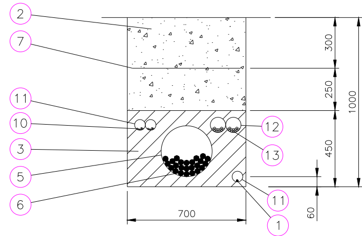
ZANJA PARA 12 CIRCUITOS BAJA TENSION EN ZONA DE TIERRA (CRUCE)
