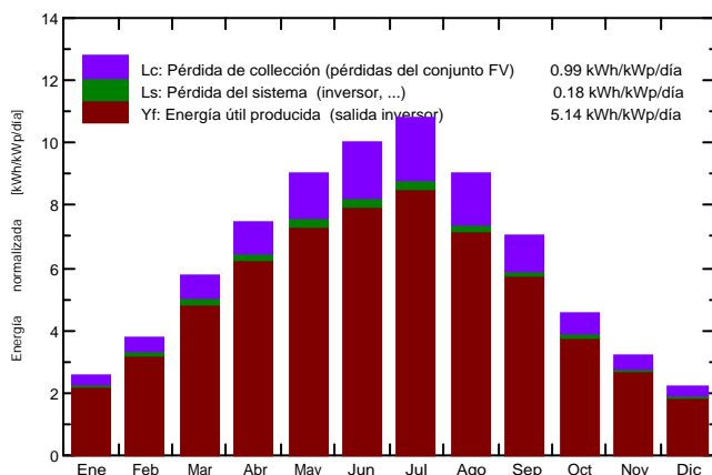
Producciones normalizadas (por kWp instalado): Potencia nominal 999 kWp
