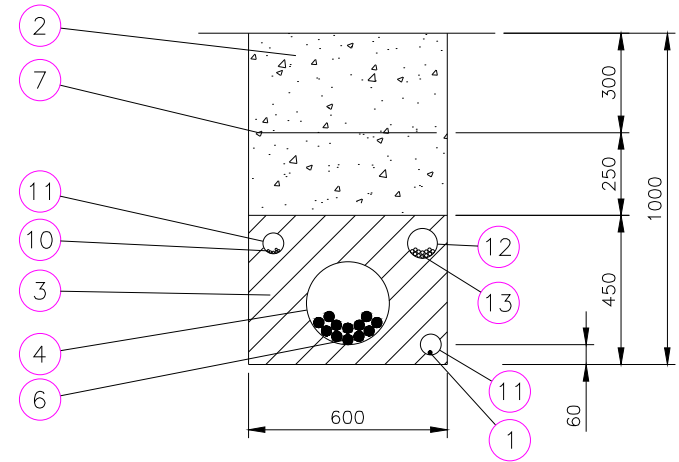
ZANJA PARA 6 CIRCUITOS BAJA TENSION EN ZONA DE TIERRA (CRUCE)
