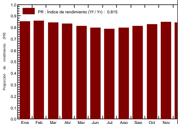
Proporción de rendimiento (PR)
