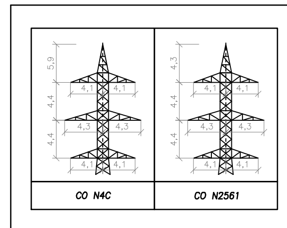
DISPOSICION DE ARMADOS ESCALA: S/E
