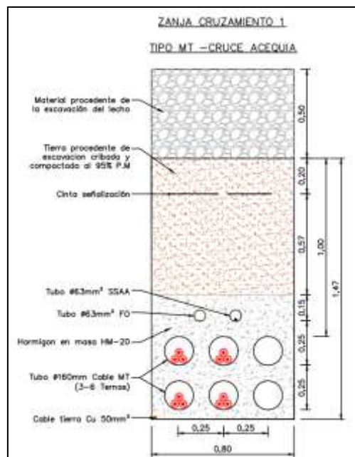
Ilustración 4: Sección zanja cruce con acequia
