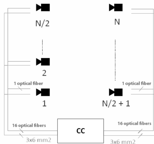
Figura 26.- Conexión general
