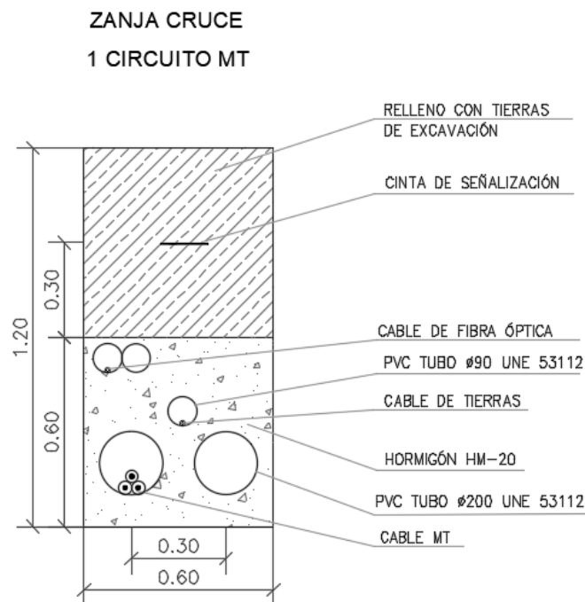
Ilustración 6. Zanja para cruce MT
