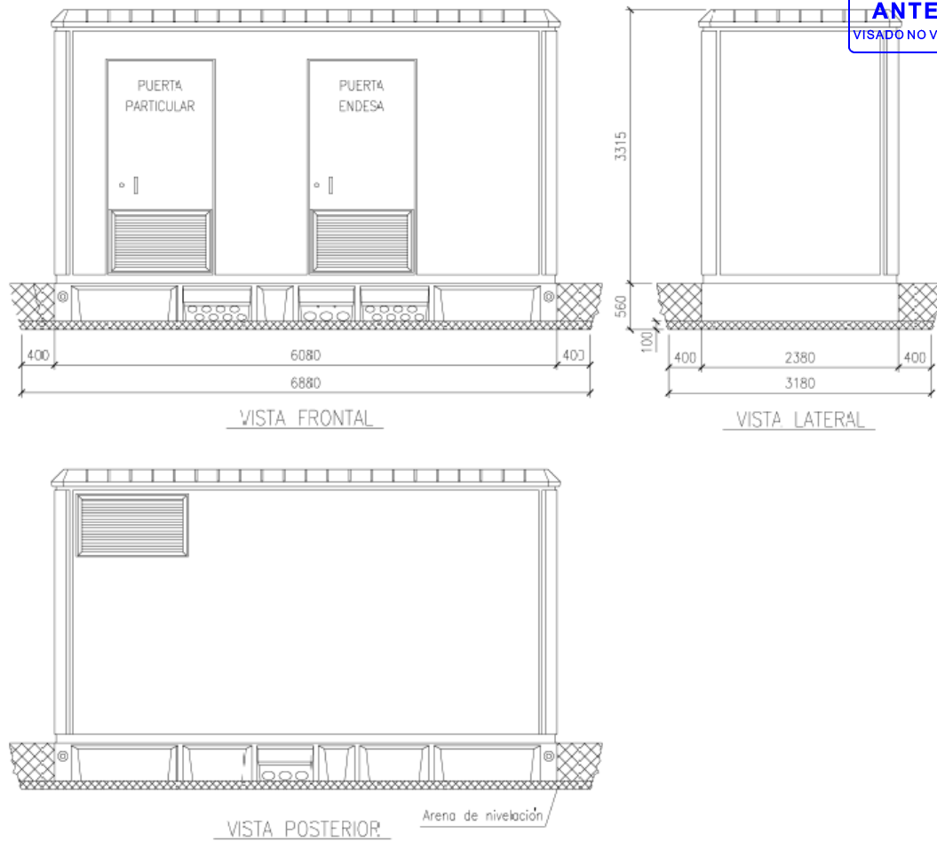
Ilustración 7. Centro de Seccionamiento. Modelo PFU-4. Fuente: Ormazabal
