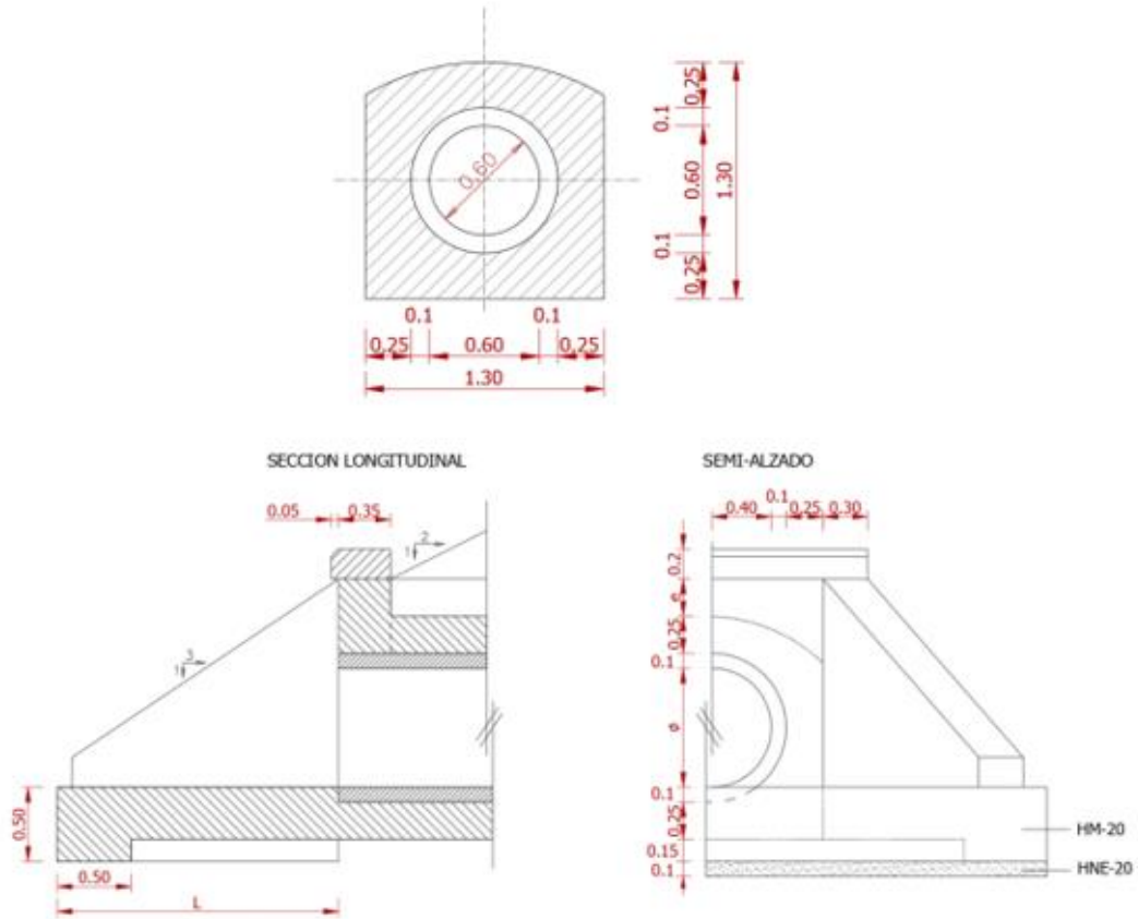
TUBERÍA DE DIÁMETRO 60 CM
