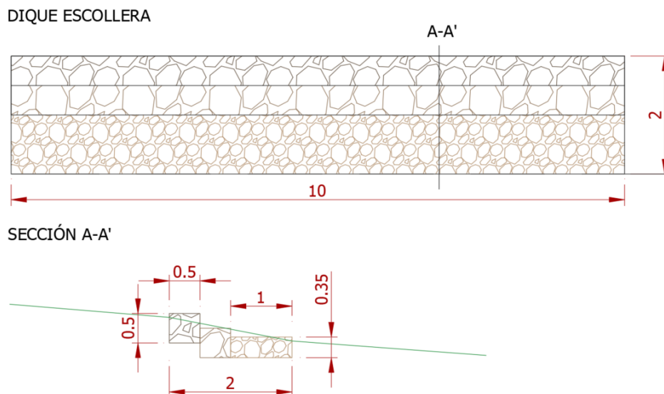
Croquis dique de escollera
