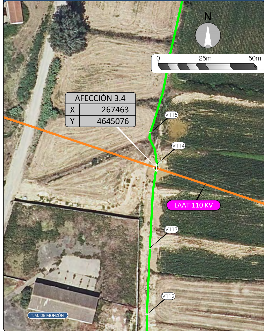
AFECCIÓN 3.4 - ESCALA 1:1.000
