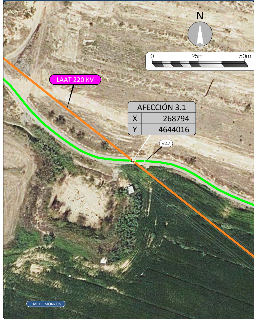
AFECCIÓN 3.1 - ESCALA 1:1.000
