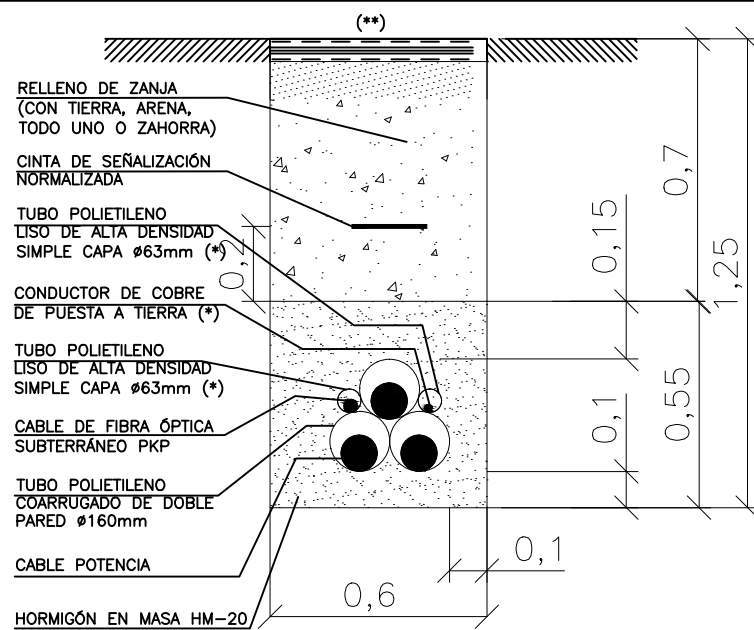
ZANJA TIPO S/C EN CRUCE
