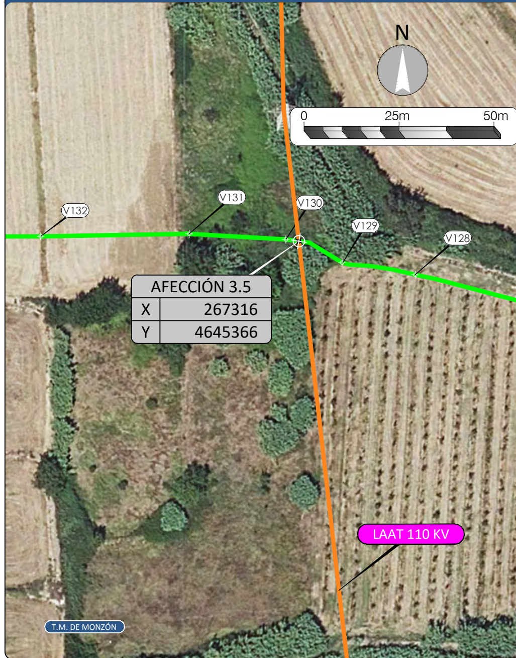
AFECCIÓN 3.5 - ESCALA 1:1.000
