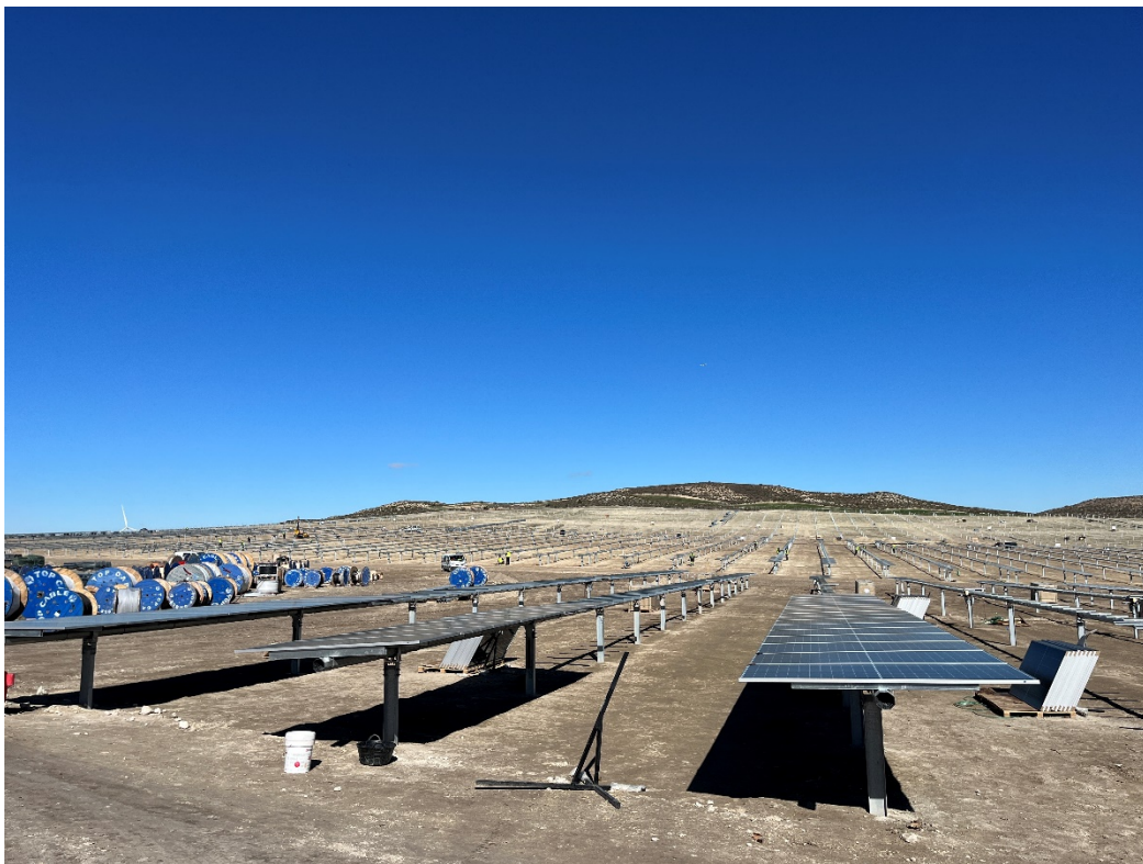
Figura 10 Montaje de los módulos fotovoltaicos
