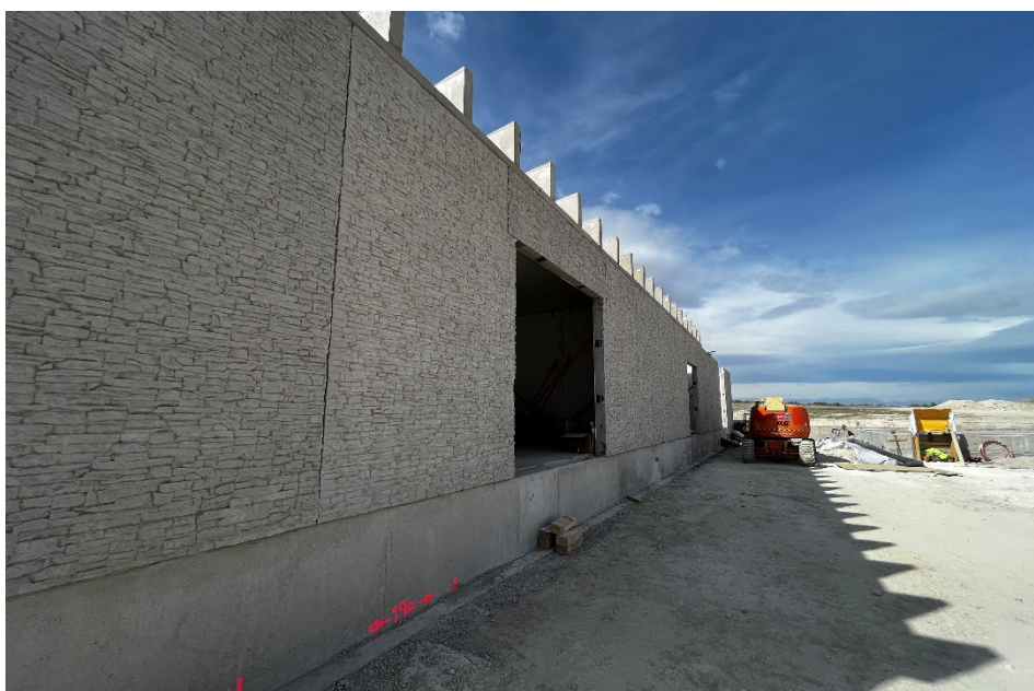
Figura 37 Montaje del edificio de control SET Cartujos
